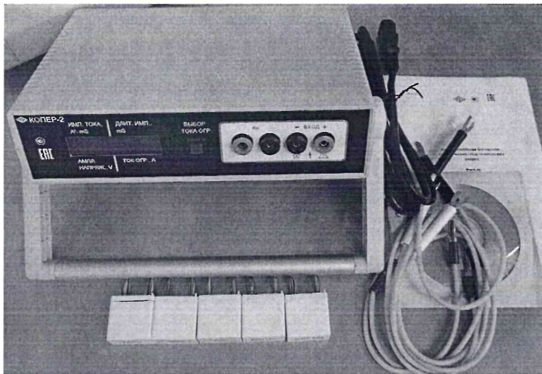
Рисунок 1.1 – Фотография общего вида прибора измерения параметров электрических средств взрывания КОПЕР-2 № 061
