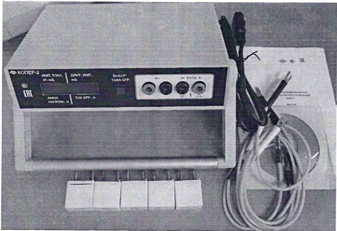
Рисунок 1.1 – Фотография общего вида прибора измерения параметров электрических средств взрывания КОПЕР-2 № 064
