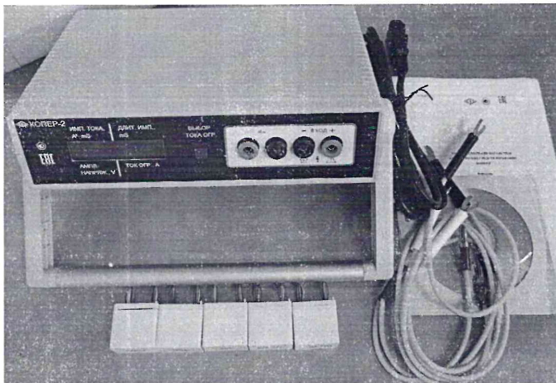
Рисунок 1.1 – Фотография общего вида прибора измерения параметров электрических средств взрывания КОПЕР-2 № 065
