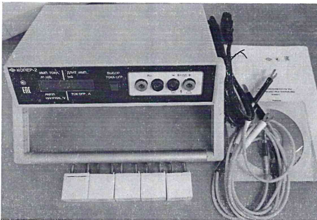
Рисунок 1.1 – Фотография общего вида прибора измерения параметров электрических средств взрывания КОПЕР-2 № 074
