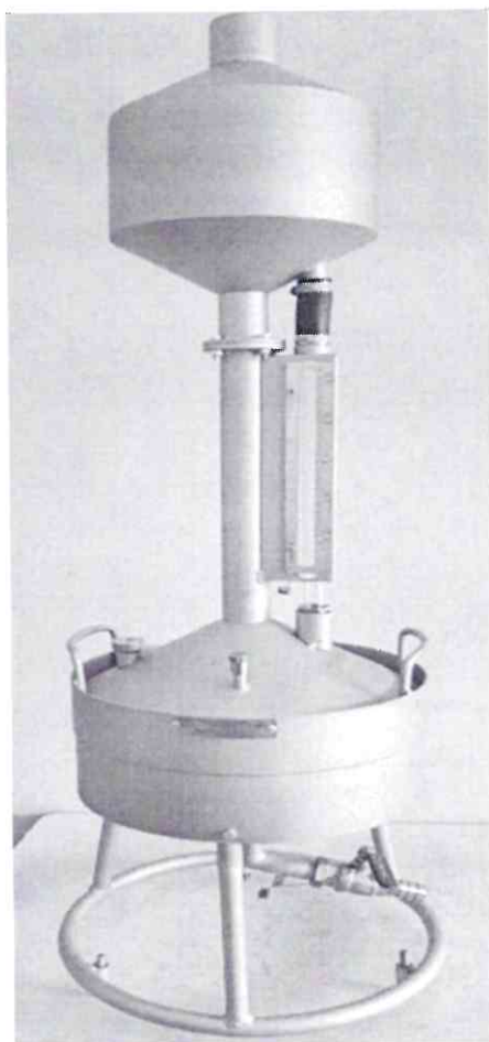
Рисунок 1.1 - Внешний вид мерника металлического эталонного М 2-го разряда 2р-10-0,05-9-11 № 044
