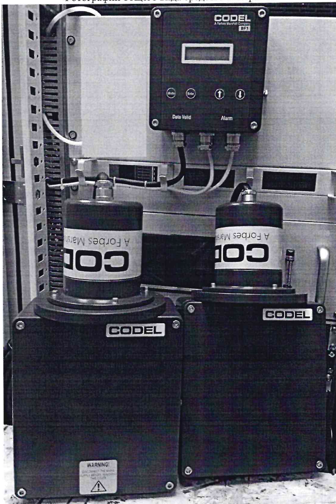
Рисунок 1.1 – Фотография общего вида. Измеритель скорости газоздушных потоков VCEM5100 № VCEM5100 – 0922 TUV SPU
