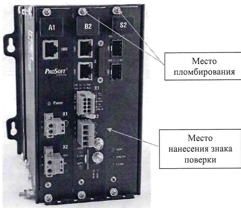
Рисунок 6 – Места пломбирования и нанесения знака поверки
