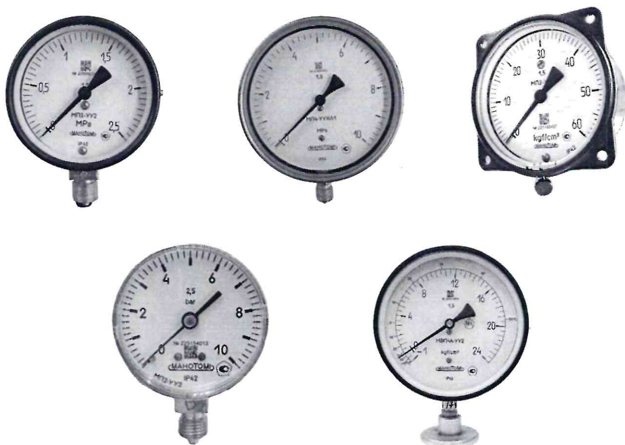
Рисунок 1 – Фотографии общего вида манометров, вакуумметров и мановакуумметров показывающих МП2-У, МП3-У, МП4-У, ВП2-У, ВП3-У, ВП4-У, МВП2-У, МВП3-У, МВП4-У
