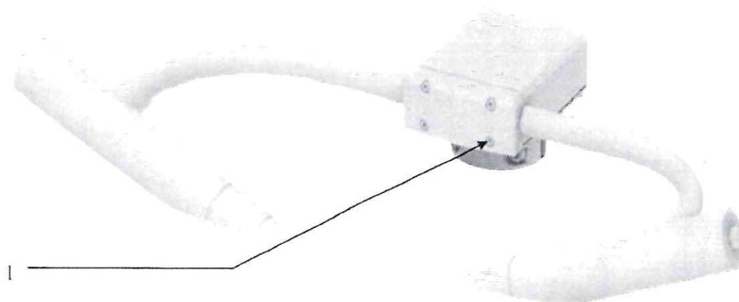
Рисунок 1 – Общий вид датчиков дальности видимости ДМДВ 1 – пломба
