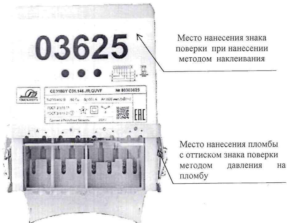
Рисунок 2.4 - Схема (рисунок) с указанием места для нанесения знака поверки на счетчик CE318BY в типе корпуса С31
