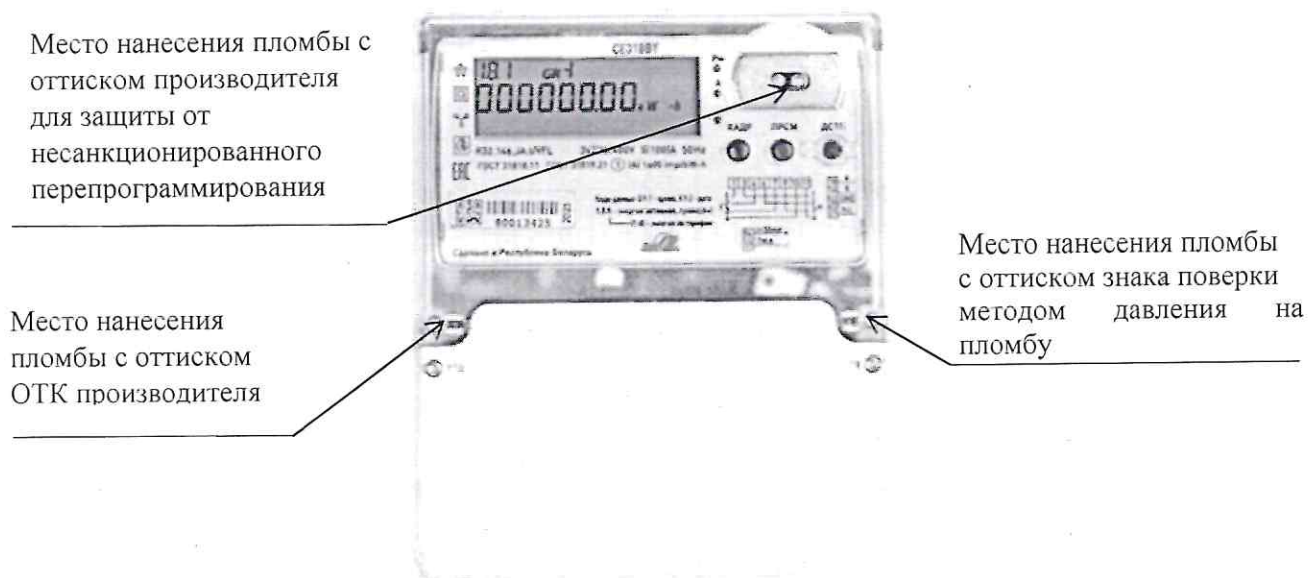
Рисунок 3.1 - Схема (рисунок) с указанием места пломбировки от несанкционированного доступа на счетчик CE318BY в типе корпуса R32
