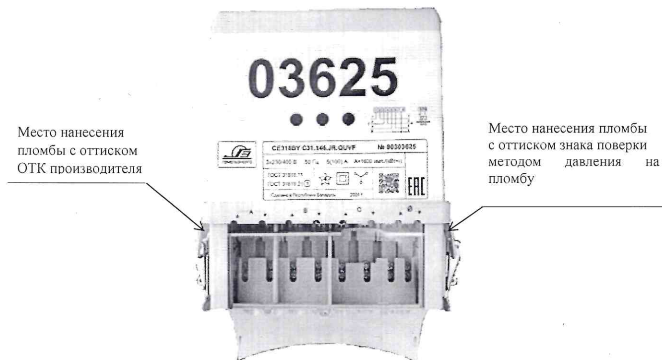
Рисунок 3.3 - Схема (рисунок) с указанием места пломбировки от несанкционированного доступа на счетчик CE318BY в типе корпуса С3
