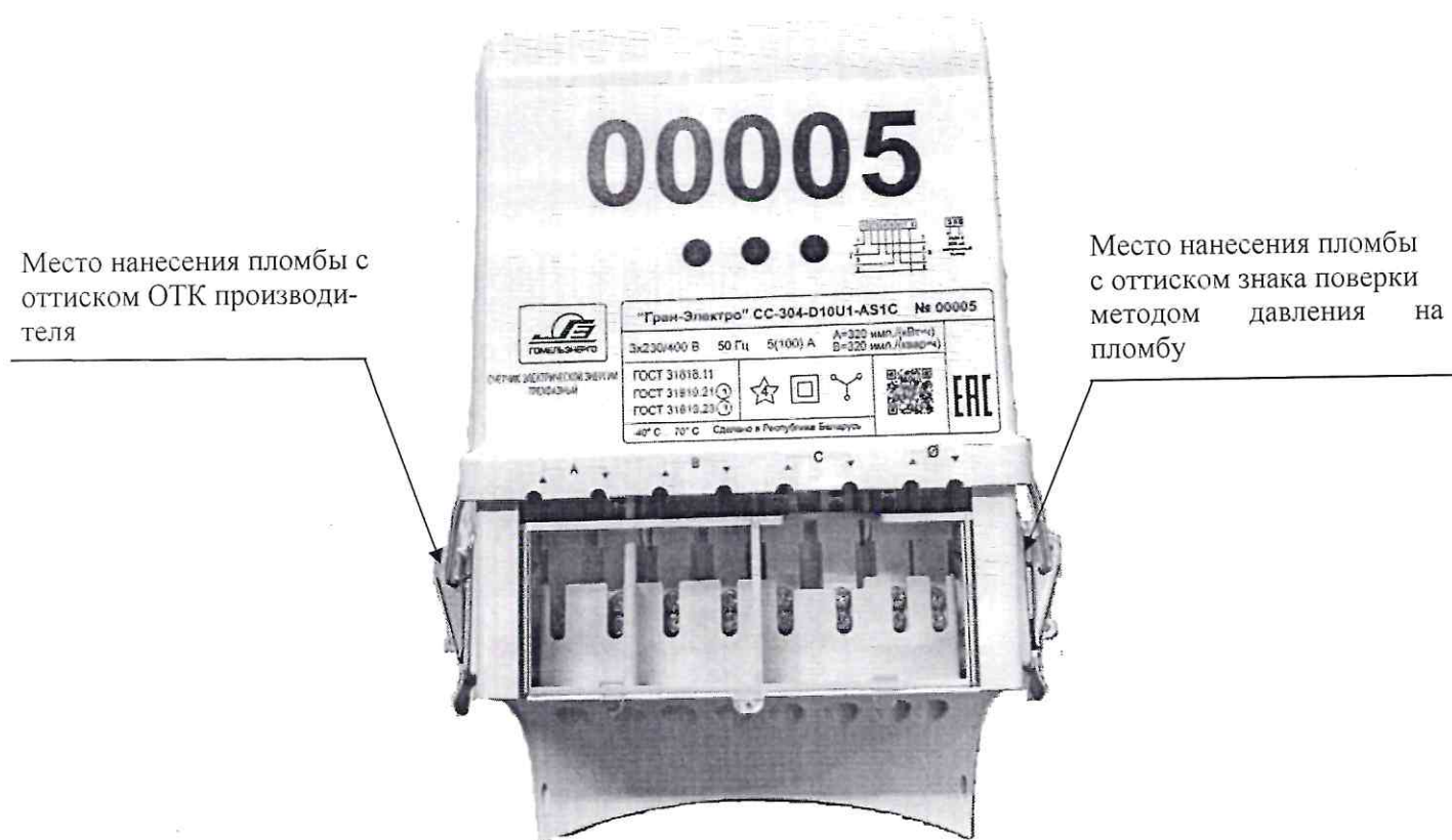
Рисунок 3.1 - Схема (рисунок) с указанием места пломбировки от несанкционированного доступа на счетчик электрической энергии трехфазный «Гран-Электро» СС-304
