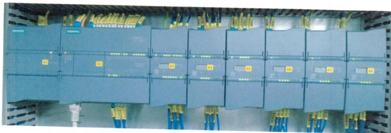
Рисунок 1.6 – Фотография контроллера программируемого SIMATIC S7-1200 с модулями ввода
