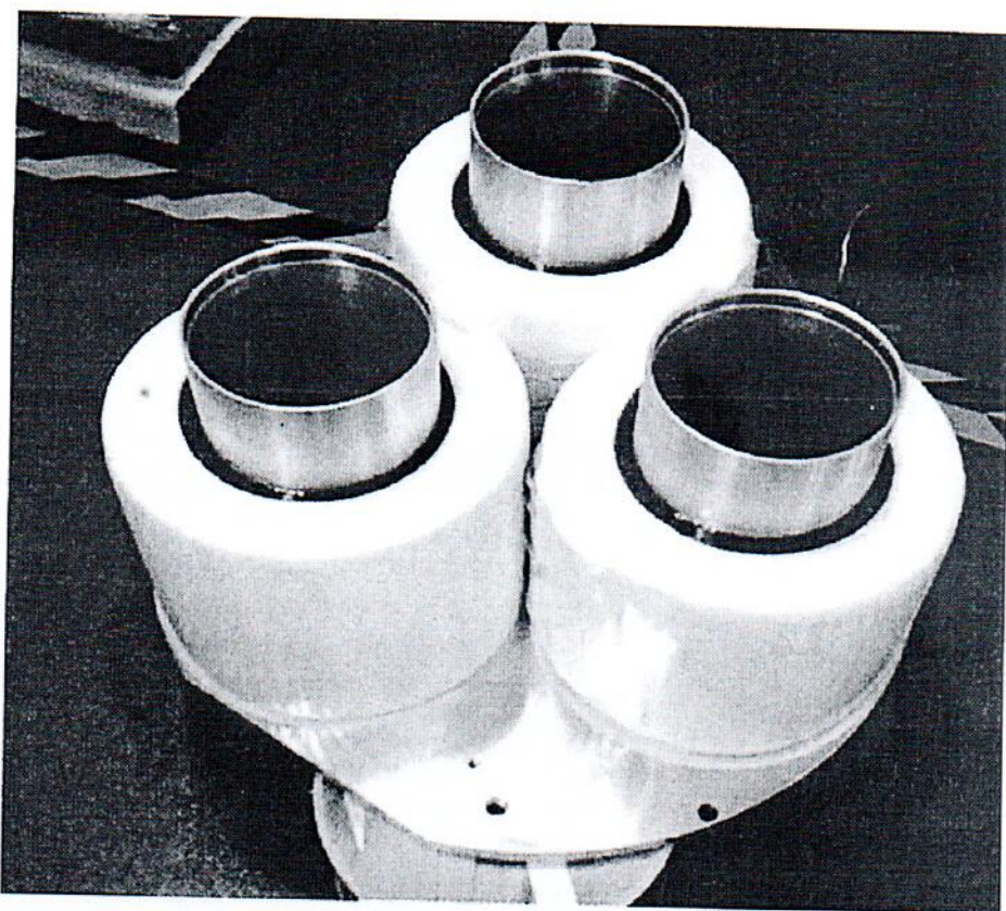
Рисунок 1.1 – Внешний вид трансформатора тока LMQB-145 № DH23010039
