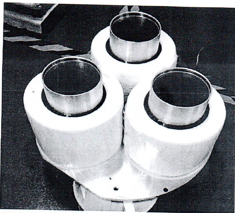
Рисунок 1.1 – Внешний вид трансформатора тока LMQB-145 № DH23010040
