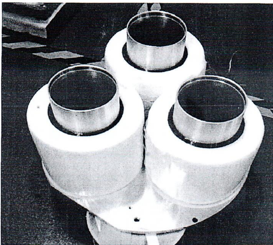
Рисунок 1.1 – Внешний вид трансформатора тока LMQB-145 № DH23010042
