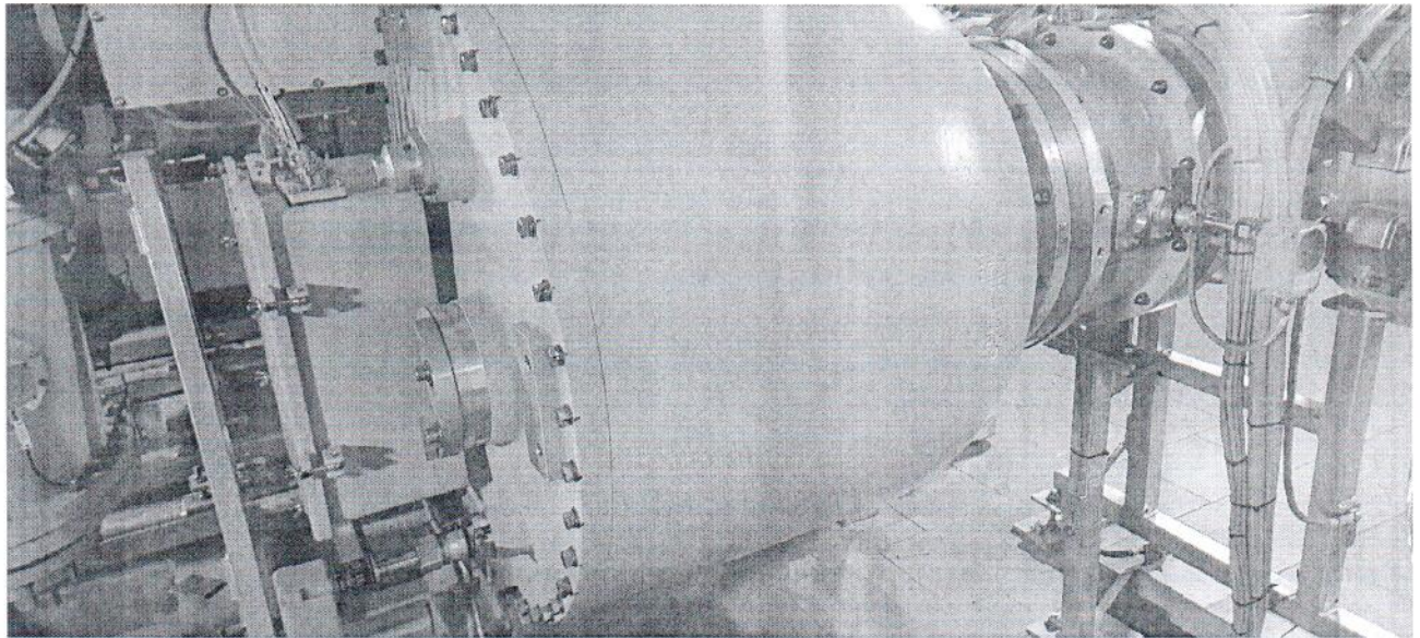
Рисунок 1.1 – Фотографии общего вида трансформатора напряжения GVT145-EL № JH23010032
