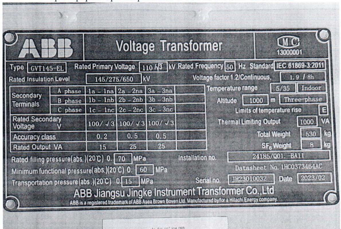
Рисунок 1.1 – Фотографии общего вида трансформатора напряжения GVT145-EL № JH23010032
