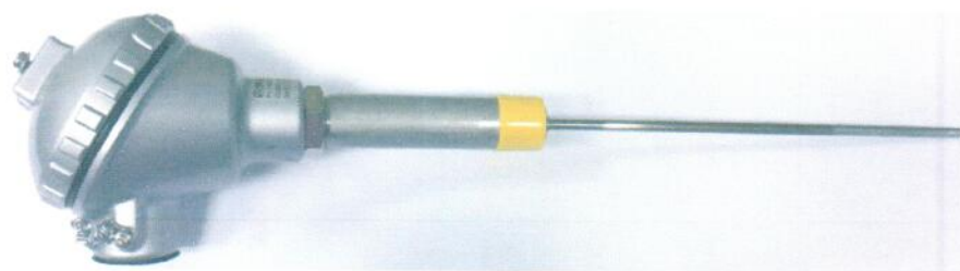
Рисунок 1.4 – Фотография преобразователя термоэлектрического ТП-Б-У
