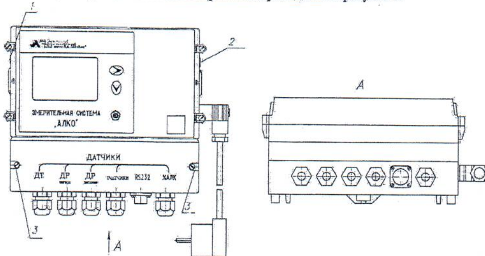
1-пломба завода-изготовителя; 2-клеимо поверителя; 3-пломба специалиста, проводившего пуско-наладочные работы Рисунок 1 - Общий вид СВ и места пломбирования
