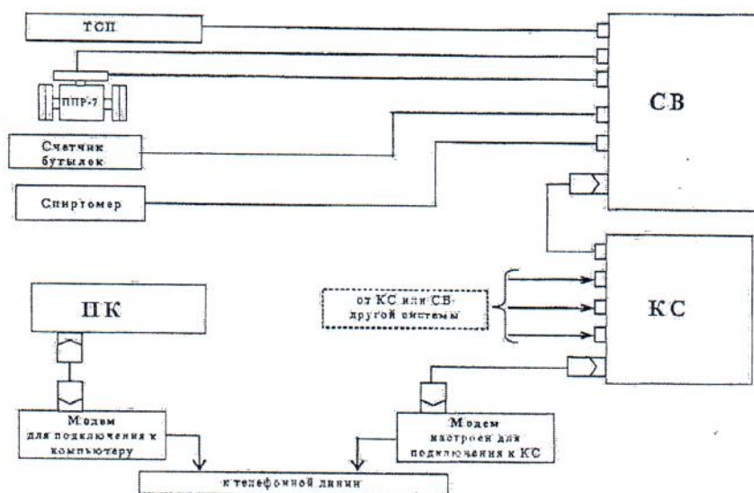
Рисунок 2 - Схема соединений составных частей системы
