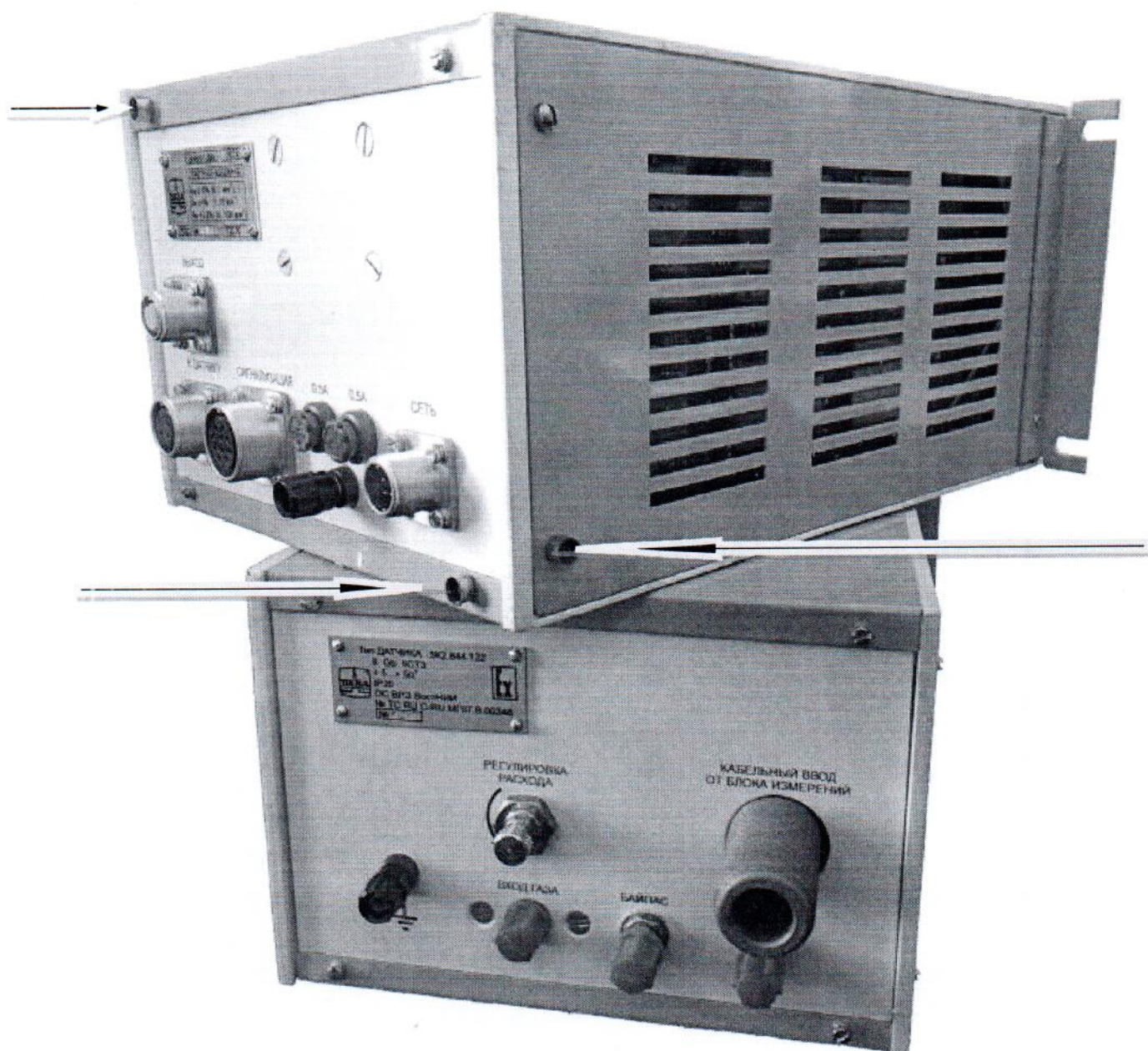
Рисунок 2 – Схема пломбировки от несанкционированного доступа гигрометра кулонометрического БАЙКАЛ-2ВМ
