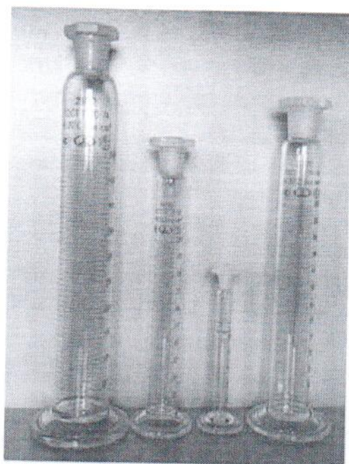
Рисунок 3 – Общий вид цилиндров исполнения 2а
