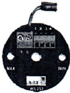
Внешний вид ИП 0304/М1
