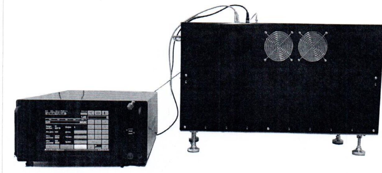
Рисунок 1 – Общий вид калибратора
