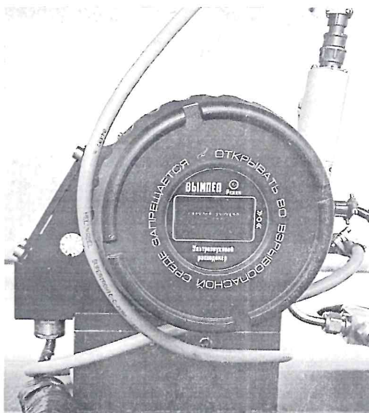
Рисунок 1.1 – Фотографии общего вида ИС УУГ
