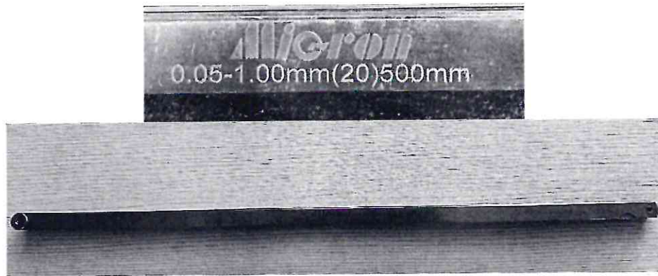
Рисунок 1.1 – Фотография общего вида набора щупов № 2023080025
