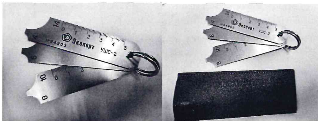
Рисунок 1.1 – Фотография общего вида универсального шаблона сварщика УШС-2 № 94903
