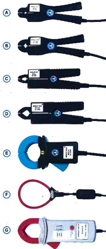
Рисунок 1.2 – Внешний вид датчиков тока А – ВФМ-ДТ-10А-П, В – ВФМ-ДТ-100А-П, С – ВФМ-ДТ-40А, D – ВФМ-ДТ-100А, Е – ВФМ-ДТ-500А, F – ВФМ-ПР-1000А, G – ВФМ-ДПТ-100А
