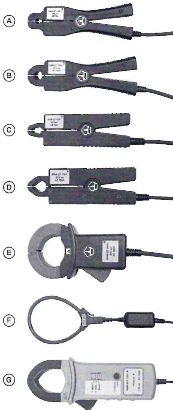
Рисунок 2 – Внешний вид датчиков тока А – ВФМ-ДТ-10А-П, В – ВФМ-ДТ-100А-П, С – ВФМ-ДТ-40А, D – ВФМ-ДТ-100А, Е – ВФМ-ДТ-500А, F – ВФМ-ПР-1000А, G – ВФМ-ДПТ-100А
