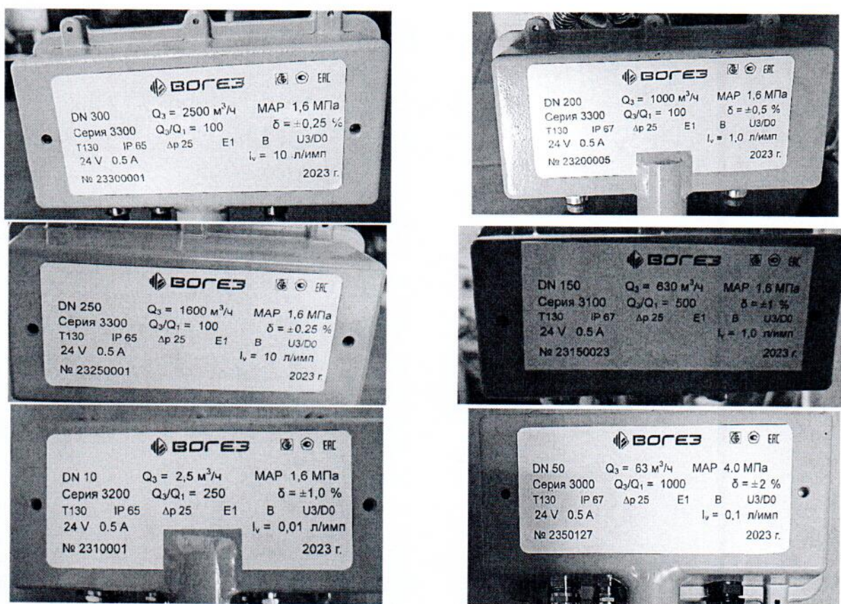
Рисунок 1.3 – Фотографии маркировки расходомеров-счетчиков электромагнитных ВИРС-М (изображение носит иллюстративный характер)
