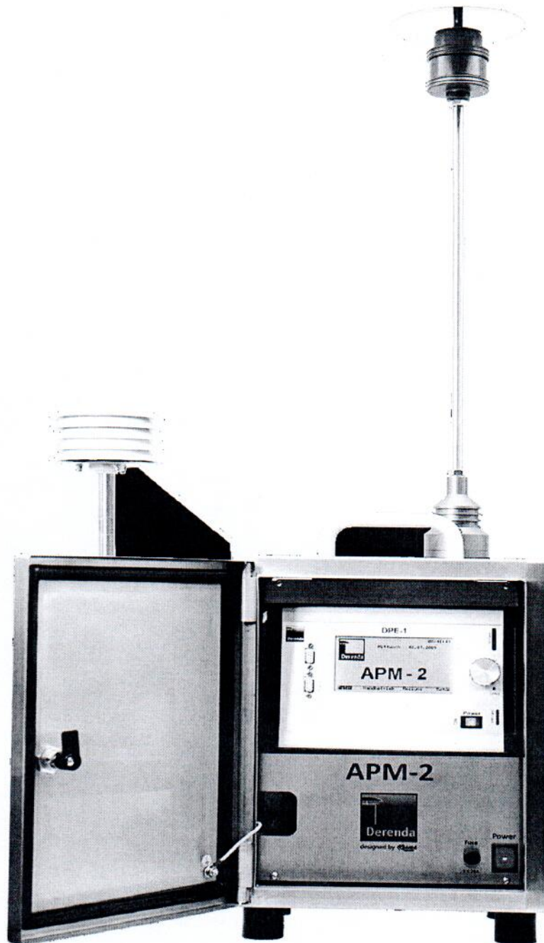
Рисунок 1.1 – Фотография общего вида анализатора пыли АРМ-2 № 20155
