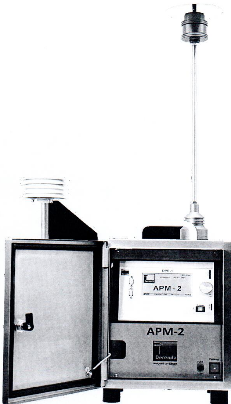
Рисунок 1.1 – Фотография общего вида анализатора пыли АРМ-2 № 20175
