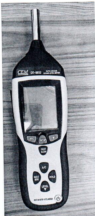
Рисунок 1.1 – Фотография общего вида измерителя уровня звука DT-8852 № 230737320
