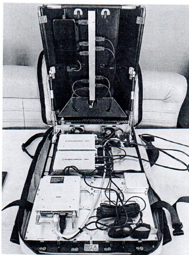
Рисунок 1.1 – Фотографии общего вида носимого измерительного комплекса для анализа параметров качества обслуживания сетей связи R&S Freerider 4 № ID 1900.6403.10-101909-AM
