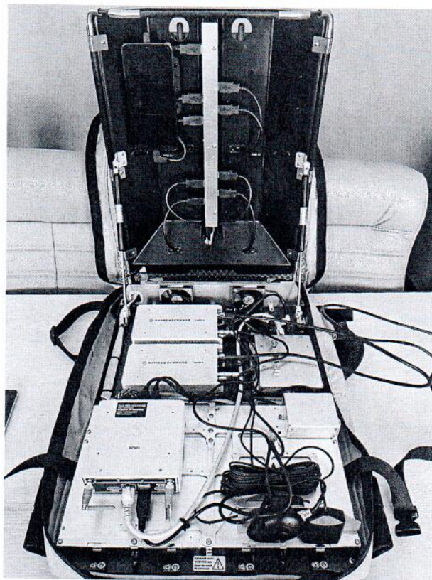
Рисунок 1.1 – Фотографии общего вида носимого измерительного комплекса для анализа параметров качества обслуживания сетей связи R&S Freerider 4 № ID 1900.6403.10-101908-jg
