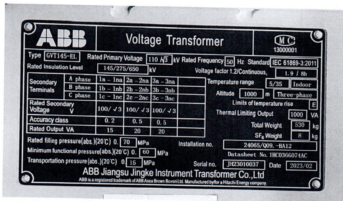
Рисунок 1.2 – Фотография маркировки трансформатора напряжения GVT145-EL № JH23010037
