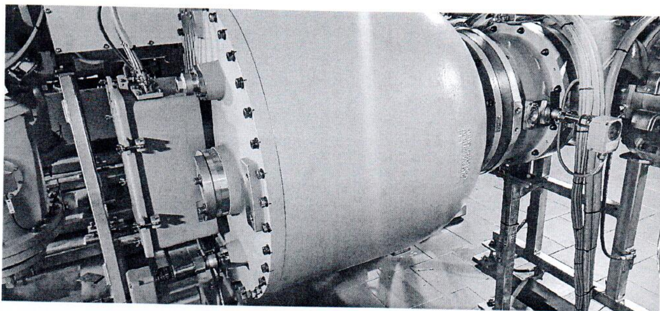
Рисунок 1.1 – Фотографии общего вида трансформатора напряжения GVT145-EL № JH23010037
