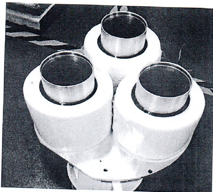
Рисунок 1.1 – Внешний вид трансформатора тока LMQB-145 № DH23010033
