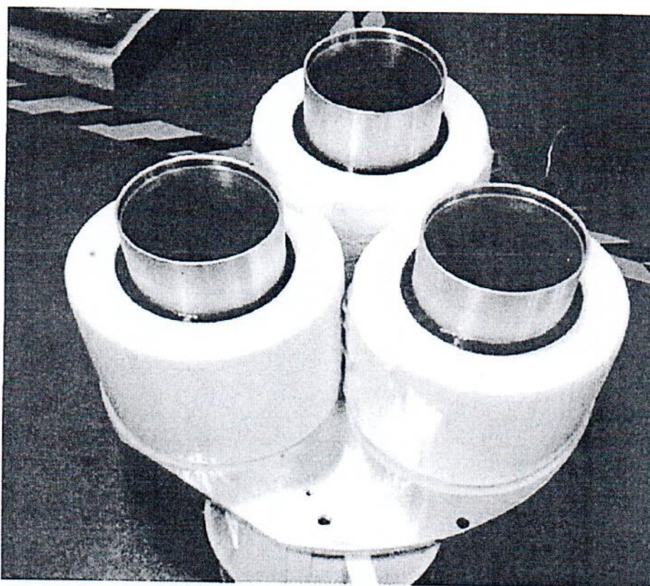
Рисунок 1.1 – Внешний вид трансформатора тока LMQB-145 № DH23010035
