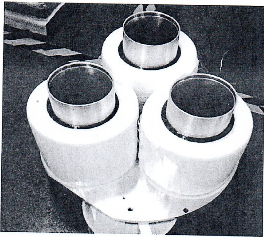
Рисунок 1.1 – Внешний вид трансформатора тока LMQB-145 № DH23010036
