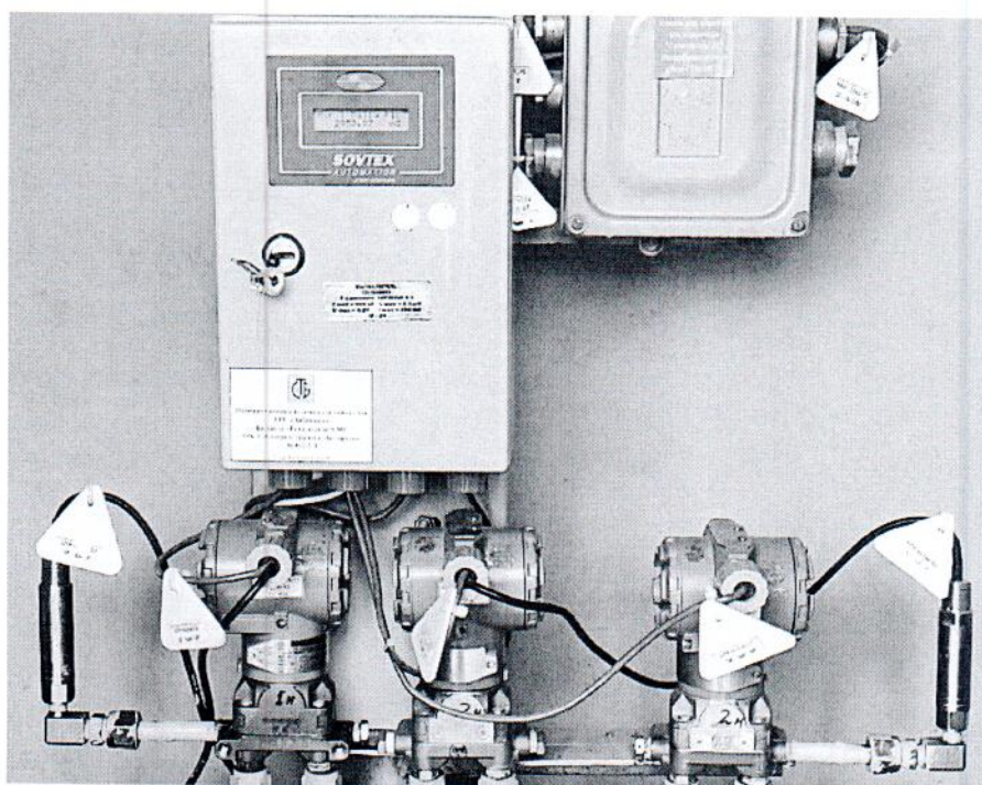
Рисунок 1.1 – Фотографии общего вида ИС УУГ
