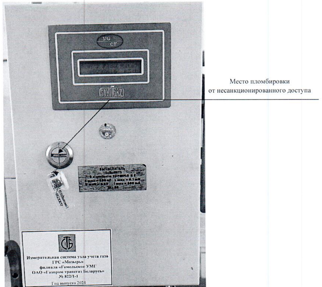
Рисунок 3.1 – Схема пломбировки от несанкционированного доступа
