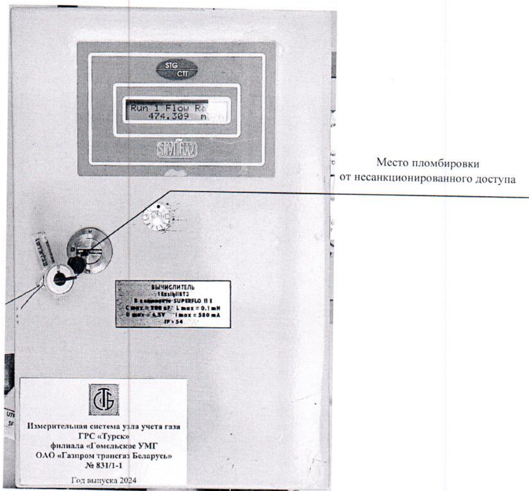
Рисунок 3.1 – Схема пломбировки от несанкционированного доступа
