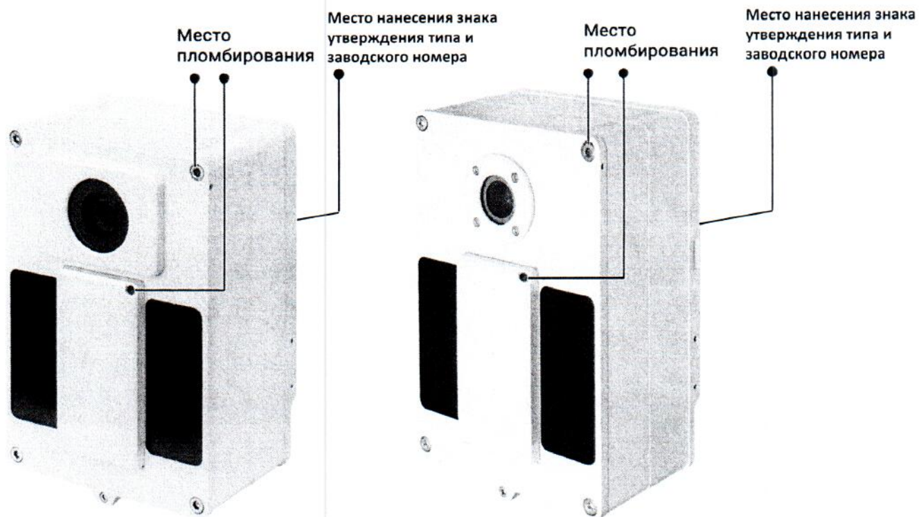
Рисунок 1 – Общий вид, места пломбирования, место нанесения знака утверждения типа и заводского номера комплекса (модификация 1) с квадратной и круглой защитной блендами
