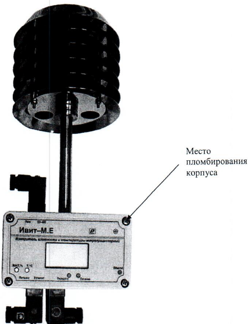
Рисунок 4 – Общий вид измерителей Ивит-М.Е конструктивного исполнения У
