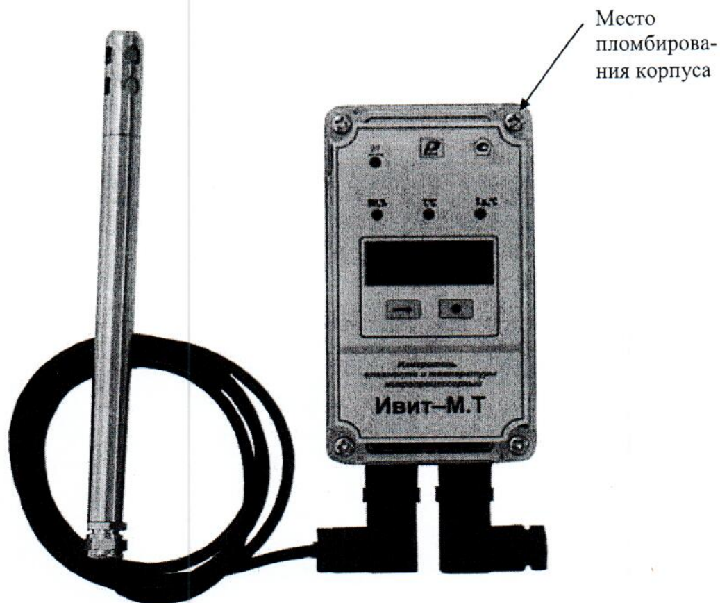
Рисунок 2 – Общий вид измерителей ИвИТ-М.Т конструктивного исполнения Н2
