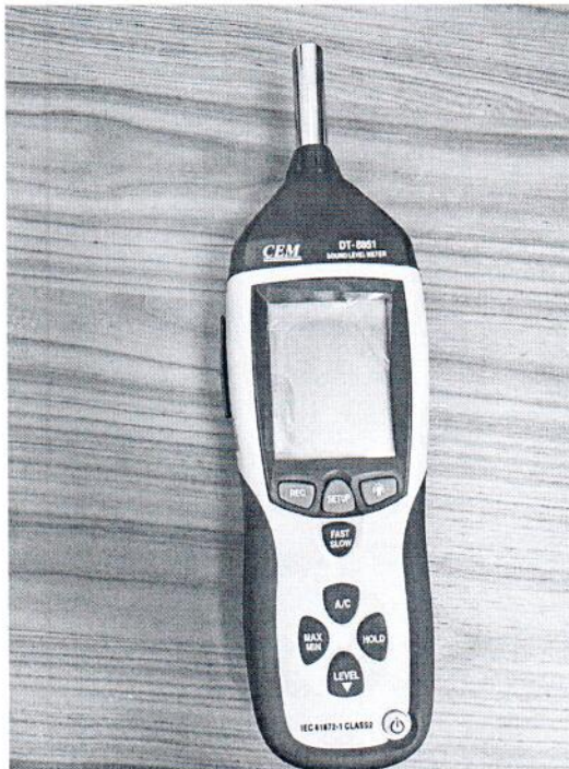
Рисунок 1.1 – Фотография общего вида измерителя уровня звука DT- 8851 № 12044632
