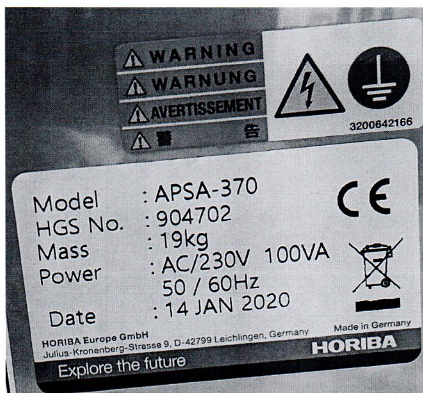
Рисунок 1.2 – Фотография маркировки анализатора диоксида серы APSA-370 № 904702
