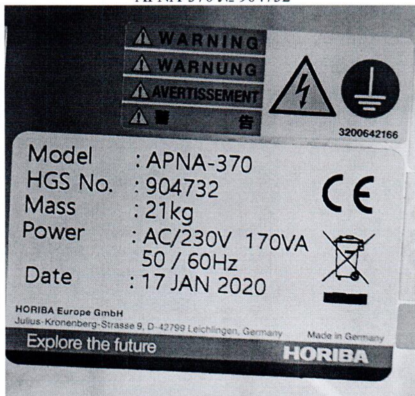
Рисунок 1.2 – Фотография маркировки анализатора окислов азота APNA-370 № 904732
