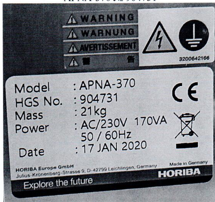
Рисунок 1.2 – Фотография маркировки анализатора окислов азота APNA-370 № 904731
