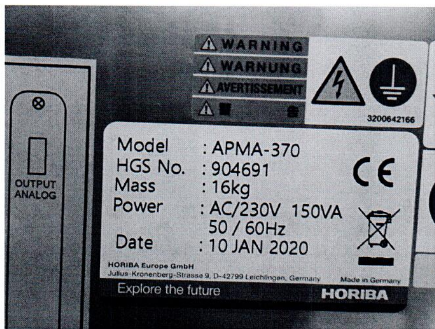
Рисунок 1.2 – Фотография маркировки анализатора оксида углерода APMA-370 № 904691
