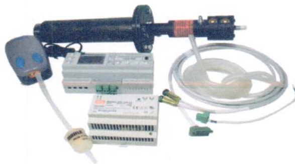
Рисунок 1.2 – Фотография анализатора кислорода ТДК-3М
