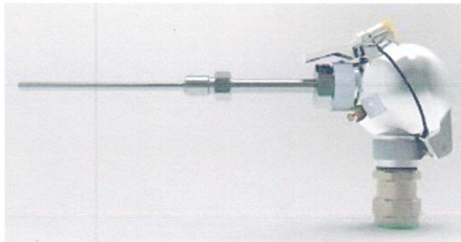
Рисунок 1.5 – Фотография термопреобразователя сопротивления ТС-Б-У
