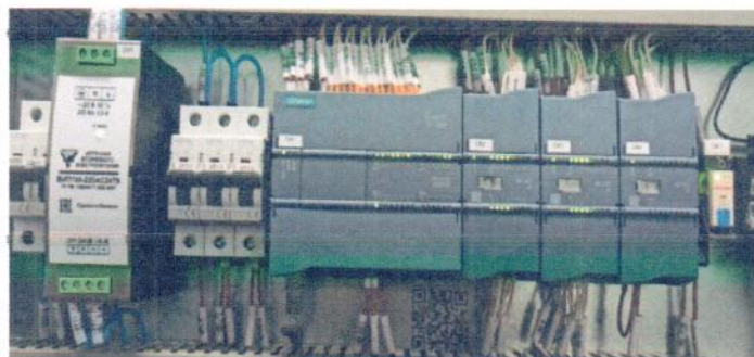
Рисунок 1.6 – Фотография контроллера программируемого SIMATIC S7-1200
