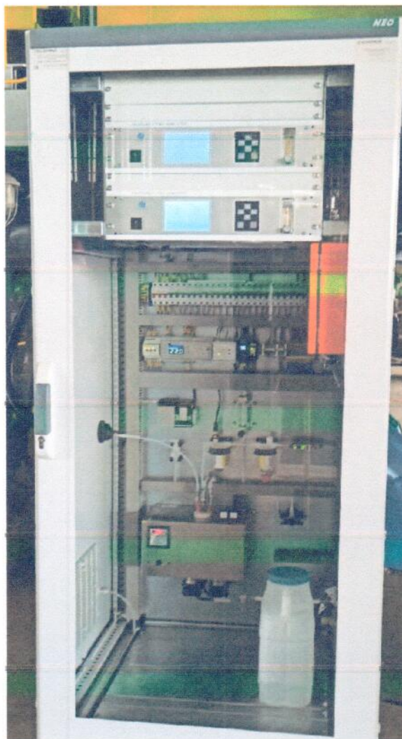
Рисунок 1.8 – Фотография шкафа газового анализа
