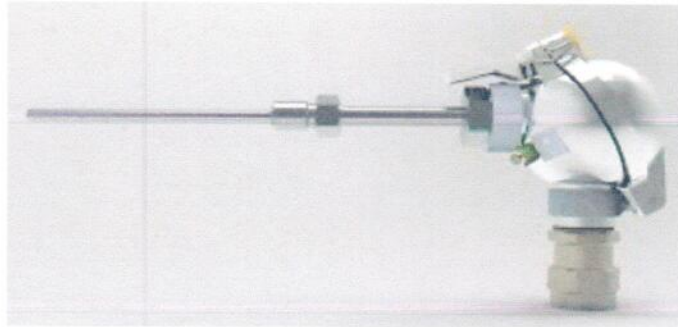
Рисунок 1.5 – Фотография термопреобразователя сопротивления ТС-Б-У
