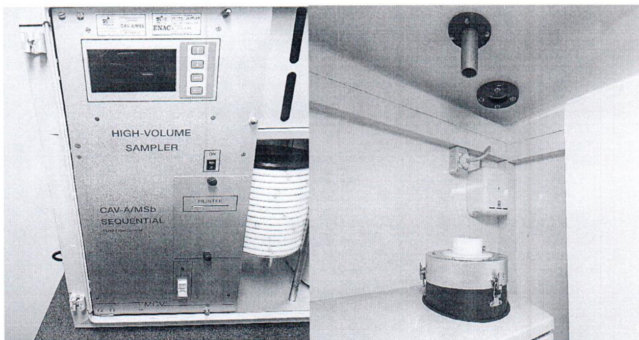
Рисунок 1.1 – Фотографии общего вида высокочастотного пробоотборника твердых частиц CAV-A/MSb № В-141/0160
