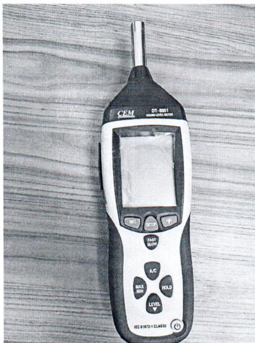
Рисунок 1.1 – Фотография общего вида измерителя уровня звука DT-8852 № 140421394
